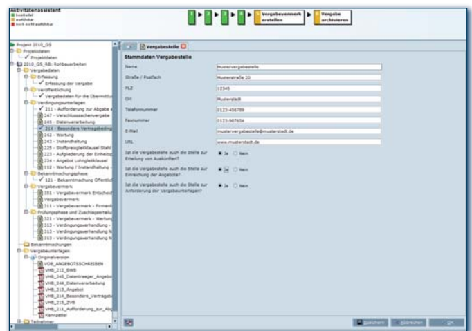
Stammdaten anlegen
