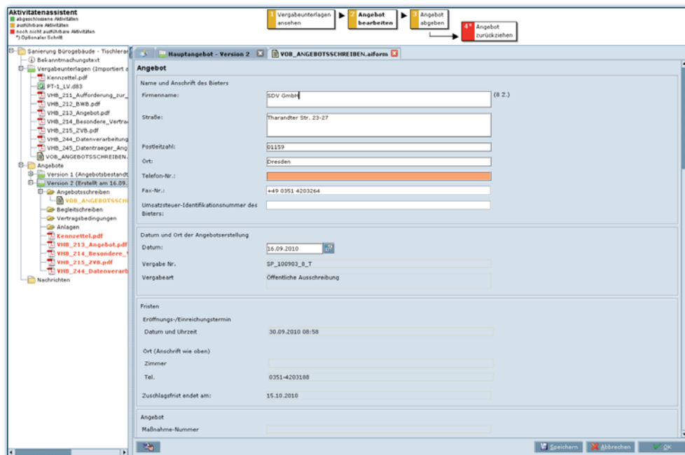
Angebot bearbeiten
