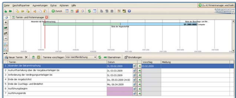
Termine anlegen
